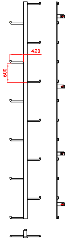
Escalera de pates Fabricada en pletina y varilla
