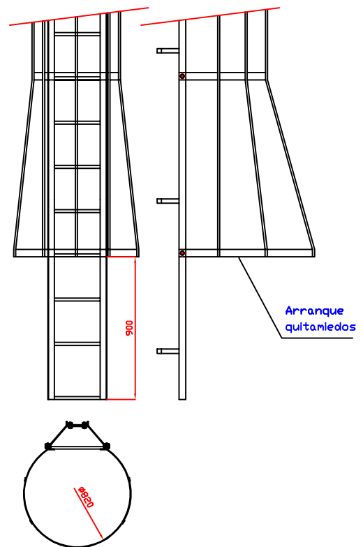
Escalera de gato con quitamiedos Fabricada en angular, varilla y pletina
