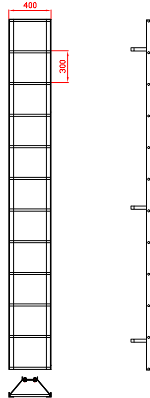
Escalera de gato Fabricada en angular y varilla
