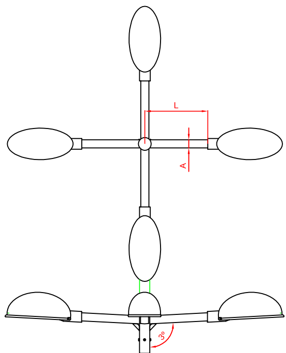
Cruceta para 4 luminarias
