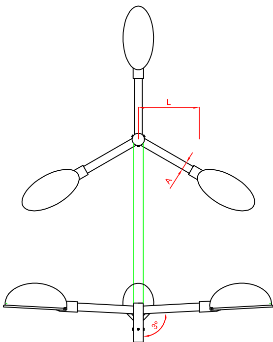
Cruceta para 3 luminarias
