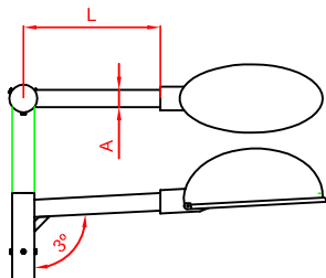
Cruceta para 1 luminaria
