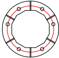
DETALLE PLACA FUSTE (Espesor=15 mm.)
