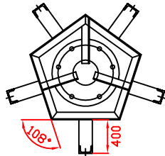
DETALLE PLACA FUSTE (Espesor=15 mm.)
